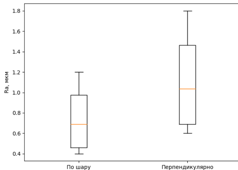
Рис. 6. Вплив напрямку різання
