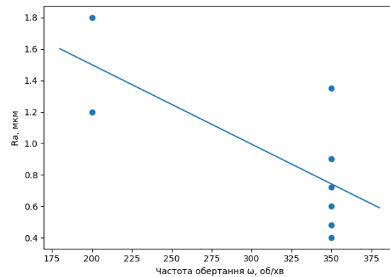
Рис. 5. Залежність Ra від частоти обертання
