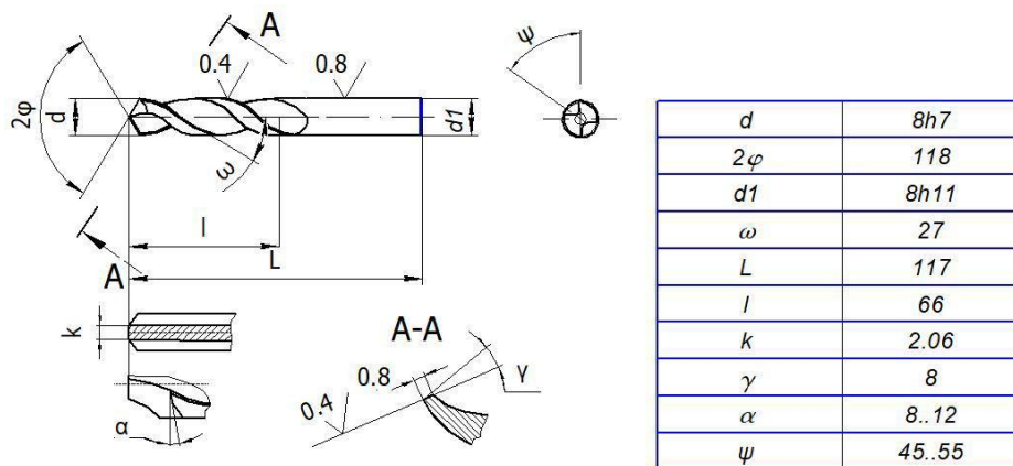
Рис. 5. Свердло Guhring 732. Дослідження проводили свердлами (рис. 4), при h = 3 мкм, h = 5 мкм, h = 7 мкм та свердлами (рис. 5) при швидкості різання V = 0,3 м/с та подачею – S = 0,4 мм/об
