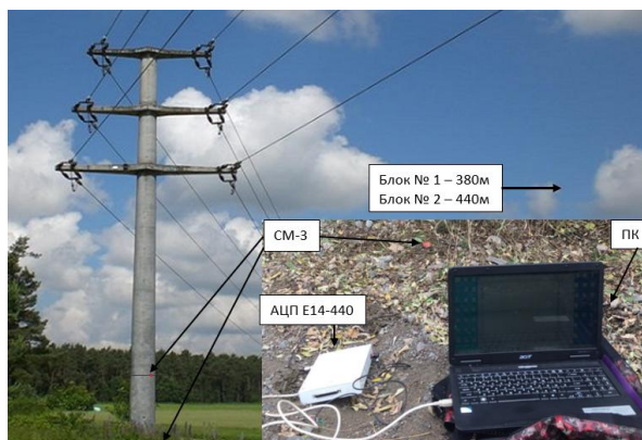
Рис. 2. Схема розташування апаратурного комплексу при дослідженні впливу масових вибухів № 1 і № 2 в умовах Коціївського гранітного кар'єру на опорі ЛЕП 330 кВ
