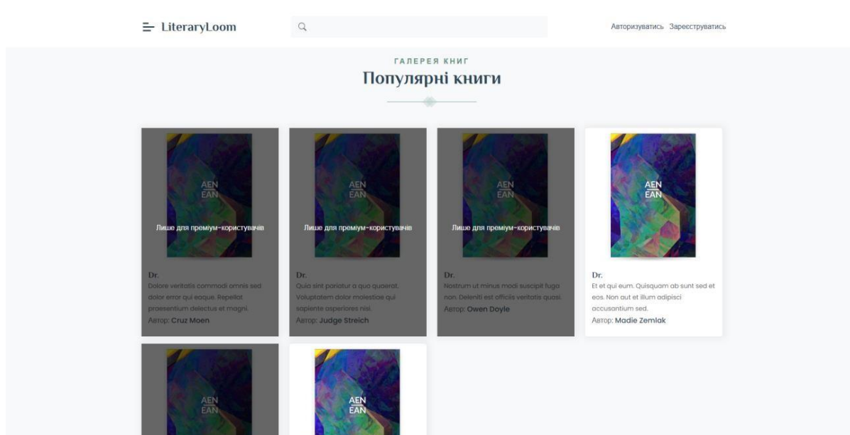
Рис. 5. Головна сторінка
