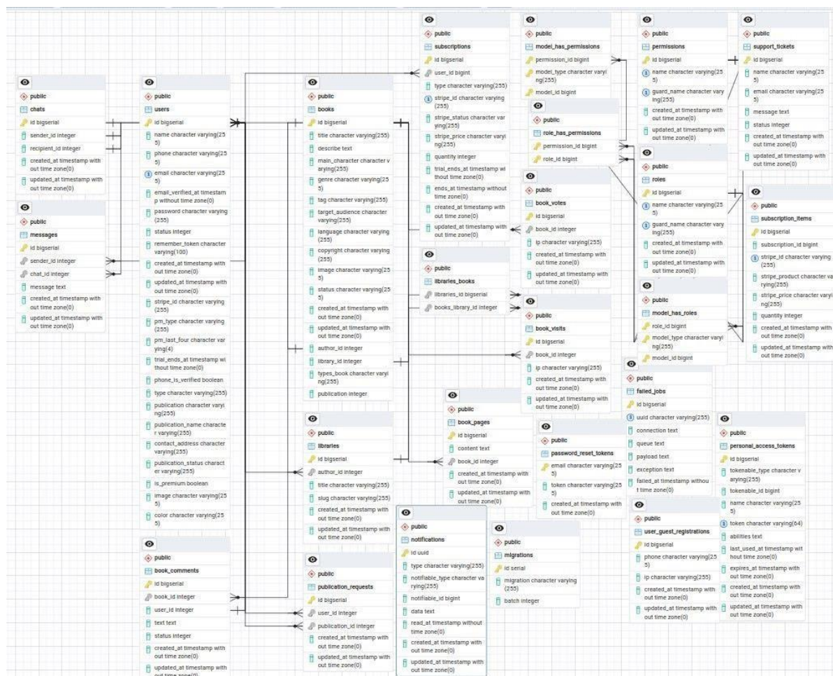
Рис. 4. Діаграма БД
